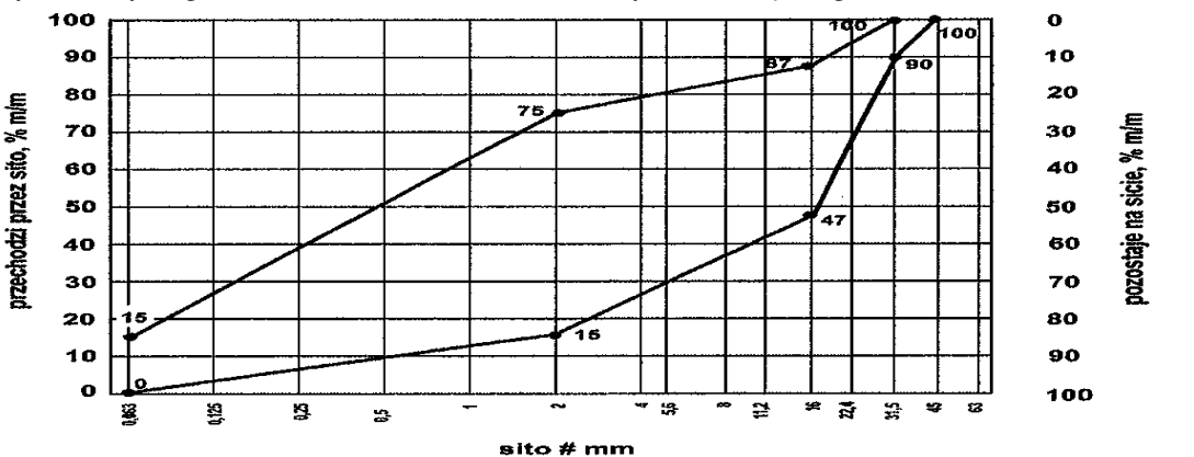
Rys. 3. Krzywe graniczne uziarnienia mieszanki kruszywa niezwiązanego 0/31,5 mm do nawierzchni
