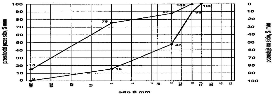
Rys. 1. Krzywe graniczne uziarnienia mieszanki kruszywa niezwiązanego 0/16 mm do nawierzchni
